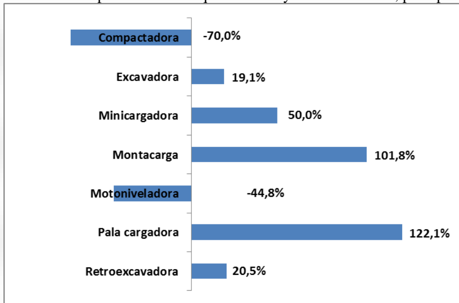
Gráfico 15: Importación de maquinaria vial y de construcción, por tipo. Variación 2018/2017
